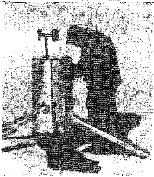
To zabawne urządzenie, które zrzucone ze spadochronu potrafi samo „stać na nogach”, (stad nazwa — konik polny) służy do przekazywania danych meteorologicznych...
