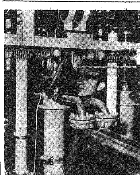
W radiostacji centralnej w Raszynie trwają prace przy montażu nowego nadajnika, surowadzanego z Czechosłowacji. Nowy nadajnik o mocy 300 KW, będzie pracował razem ze starym nadajnikiem, którego moc wynosi 200 KW. Dzięki tak zwiększonej mocy (500 KW) radiostacja w Raszynie będzie nadawała program bez przerwy południowej, znacznie zwiększając swój zasięg.
