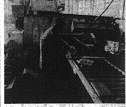
Nowy zakład obróbki marmuru w Bolesławicach. Na zdjęciu fragment linii waformera. Fot. A. Pęczalski.
