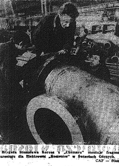
Brigada Stanisława Korusa i „Chemaru” montują fragment rurociągu dla Elektrowni „Kosminco” w Świerżach Górnych.
