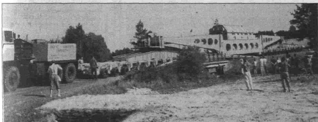
Specjalny zestaw transportowy (jedyne w Polsce) umożliwiający przewóz ładunków ultraciężkich, a w szczególności transformatorów o ciężarze do 300 ton. Zestaw składa się z ciągnika marki „willem” o uciagu na haku 1000 ton i dwóch zestawów przyczep drogowych marki „cometto”, które łącznie mają 28 osi. Umożliwia to bardzo korzystne rozłożenie nacisku na jezdnię, w tym mosty.
