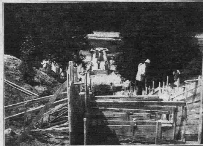
Budowa schodów prowadzących do pomostu nad wodą.
