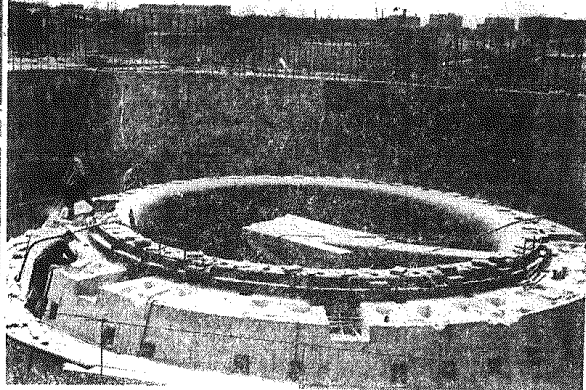
Prace przy obudowie wlotów turbin.
