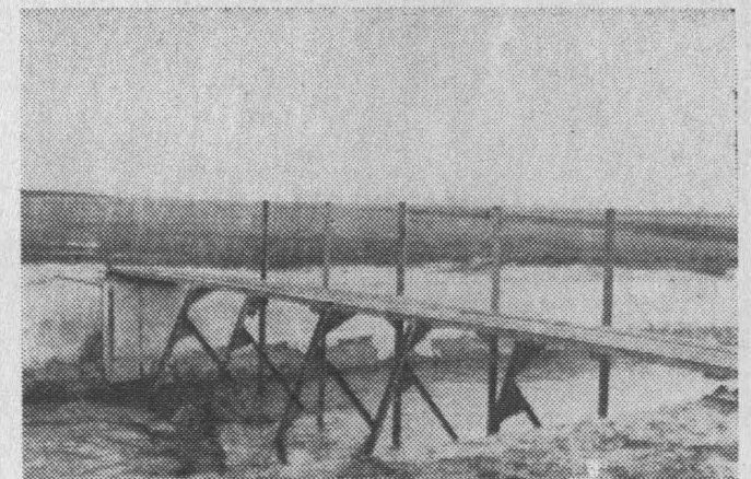
Obiekt melioracyjny Wschodnia — Brody. Jar korbowy na „młynówce”. Obiekt oddany będzie do użytku w 1965 r.
