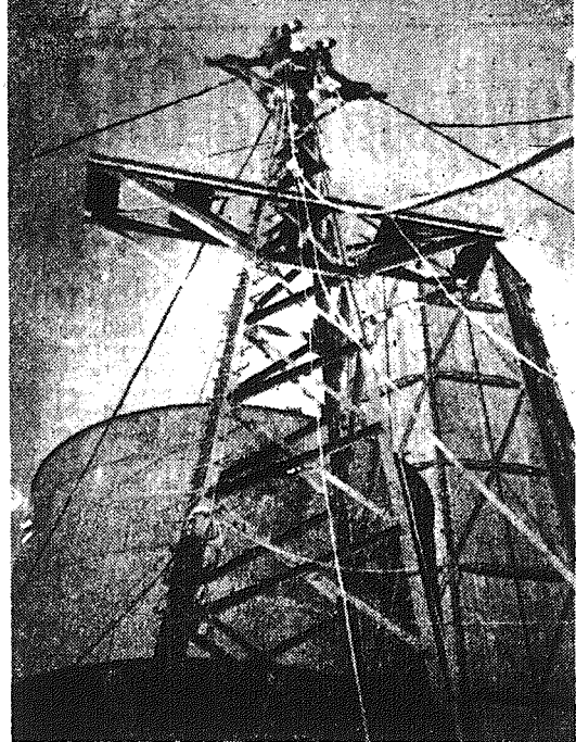
Budowa kolejki linowej między kopalniami „Chrobry”, „Mieszko”, „Viktoria” i „Thorez” w Walbrzychu ma na celu usprawnienie transportu różnych typów węgla wg jakości do odpowiednich zakładów koksowniczych.
