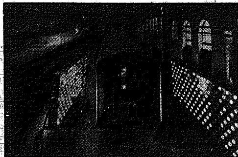
Fabryka Wagonów Dunakeszi (Węgry) produkuje wagony z części prefabrykowanych. Metoda te opracował naczelny inżynier fabryki Józef Györfi, który przebiegając w Polsce zapoznał się z naszymi metodami produkcji taboru kolejowego. Na zdjęciu: suszenie pomalowanych wagonów promieniami podczerwonymi. Fot. — CAF.
