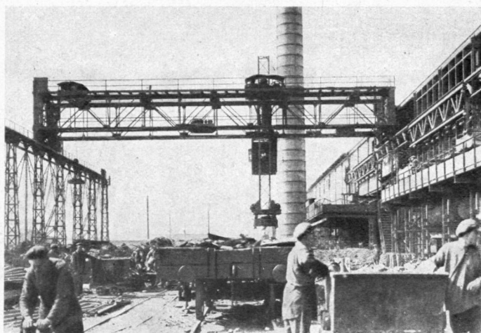
Suwnica placowa 7,5 ton. z wózkiem 4 ton. magnesowym Pont roulant de 7,5 tonnes à mitraille 7,5 tons magnet crane Magnetkran
