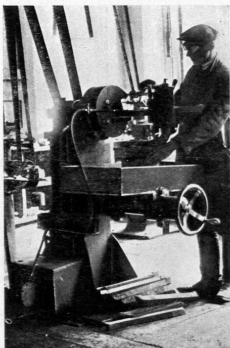
Szlifierka o kadłubie i częściach spawanych. Machine à meuler avec corps et parties soudés. Grinding machine with welded body and parts. Schleifmaschine in gänzlich geschweisster Ausführung.
