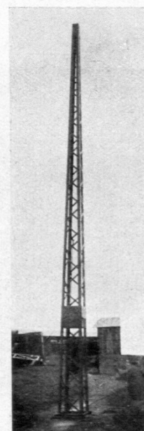
Słup stalowy dla tramwajów elektrycznych Poteau en acier pour tramways électriques Steel poles for tramways in coal district Stahlmast für elektrische Strassenbahnen
