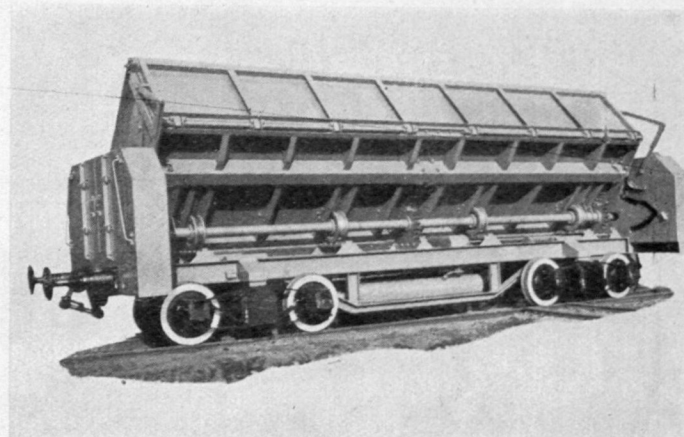
Wagon samoopróżniacz Wagon basculant Self-discharging wagon Selbstentlader.
